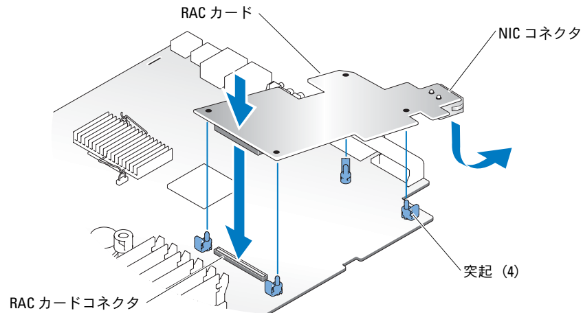
図 2. RAC カードの取り付け
